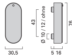
Dornrosette mit Dornloch und Verdeck, senkrecht DRS Rose with aperture and swing cover (vertical) DRS
