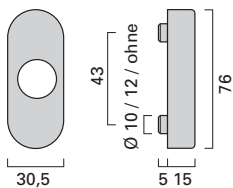
Dornrosette mit Dornloch und Verdeck, waagrecht DRW Rose with aperture and swing cover (horizontal) DRW
