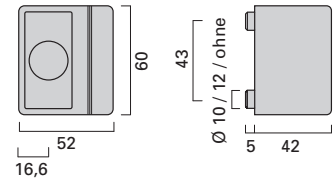
Schließanlagen-Beschlag SA Window rose to suit Euro-profile cylinder SA
