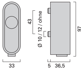
Fenster-Rosette, verschließbar, FV Lockable window rose FV
